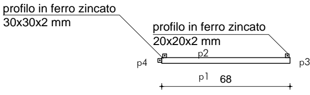
pianta
