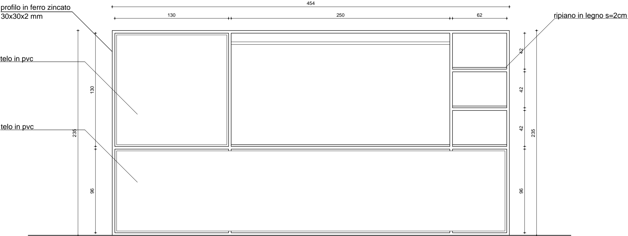
prospetto frontale 1:25
