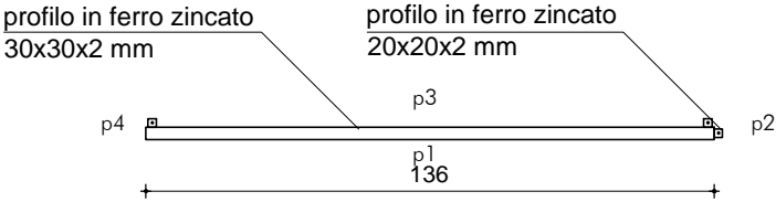
pianta
