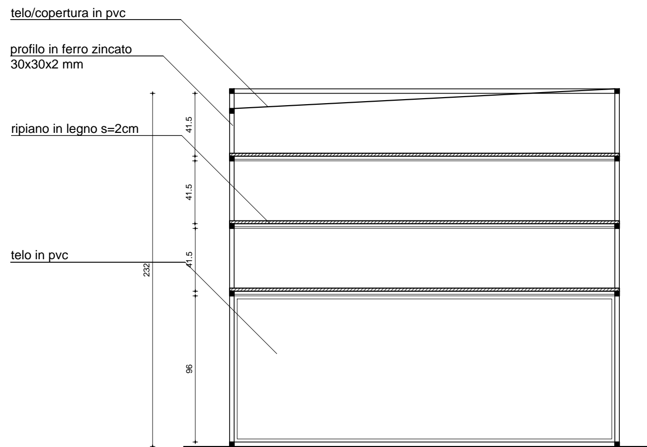
sezione A-A 1:25
