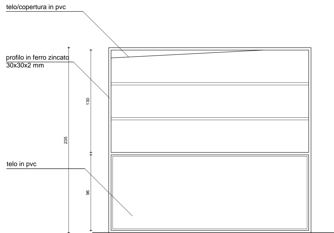
prospetto laterale sinistro 1:25
