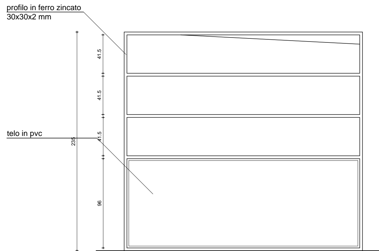
prospetto laterale destro 1:25
