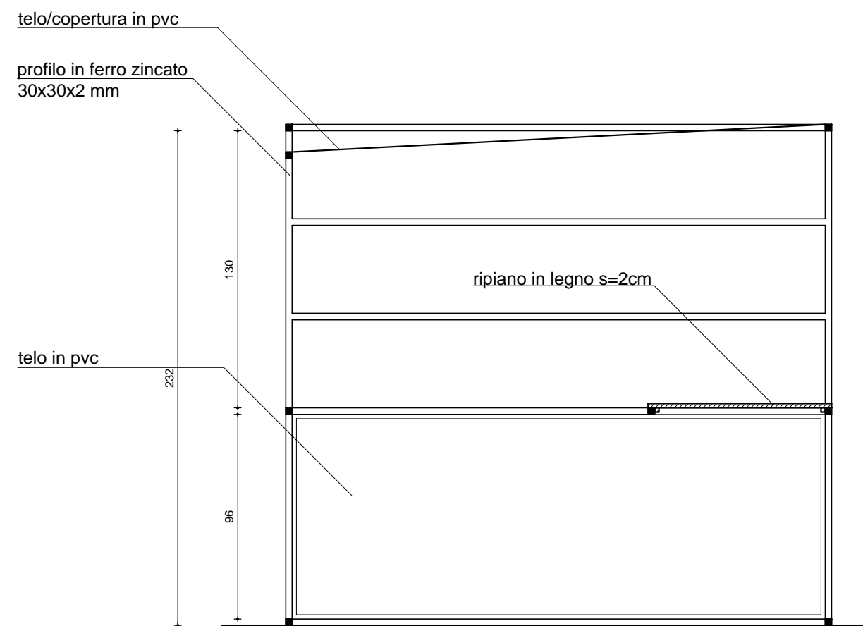
sezione B-B 1:25
