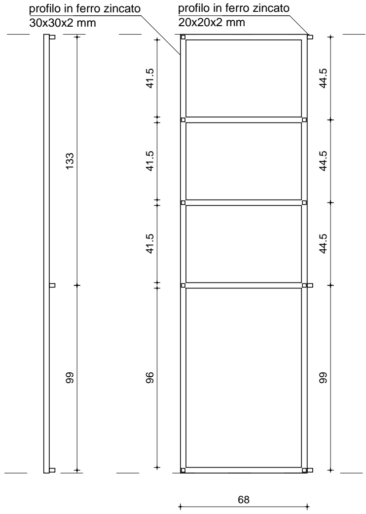
prospetto 2
