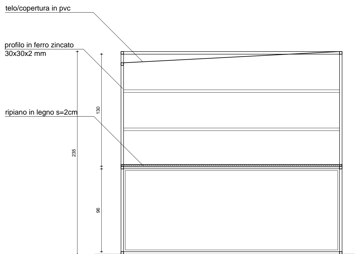
sezione C-C 1:25
